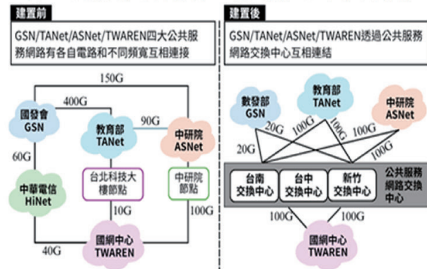
圖 5 公共服務網路交換中心建置前後之公部門網路架構
