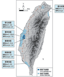
圖 7 全臺顯著地層下陷面積及最大下陷速率
